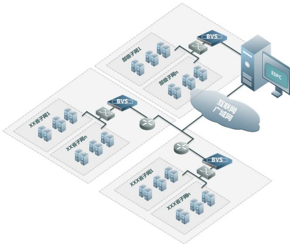
图 3.9 NSFOCUS BVS 分布式部署架构图
