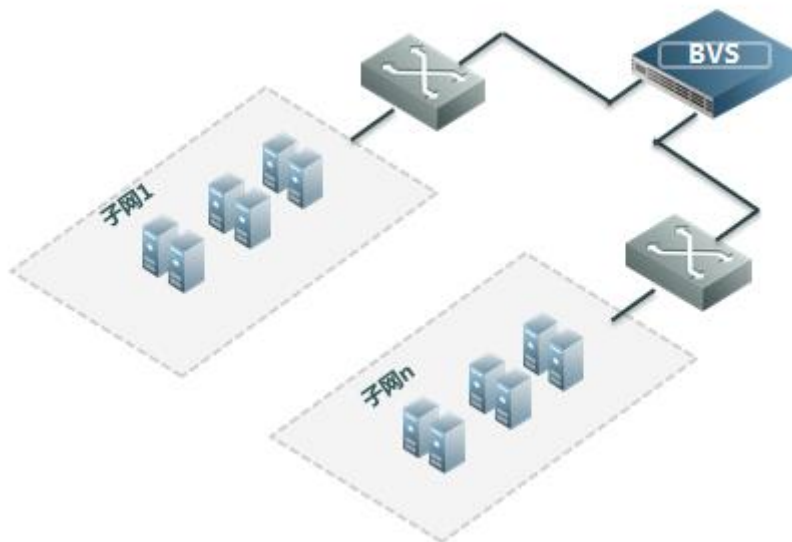
图 3.7 NSFOCUS BVS 单机多网口多子网接入
